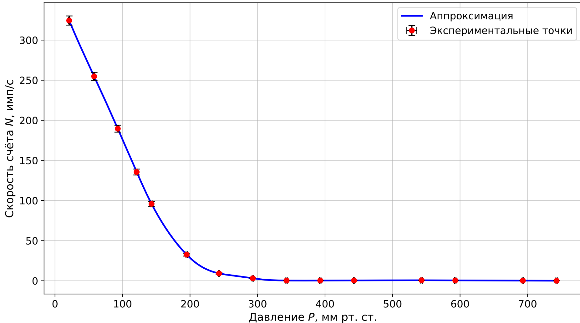
Зависимость скорости счёта от давления (линейный масштаб)
